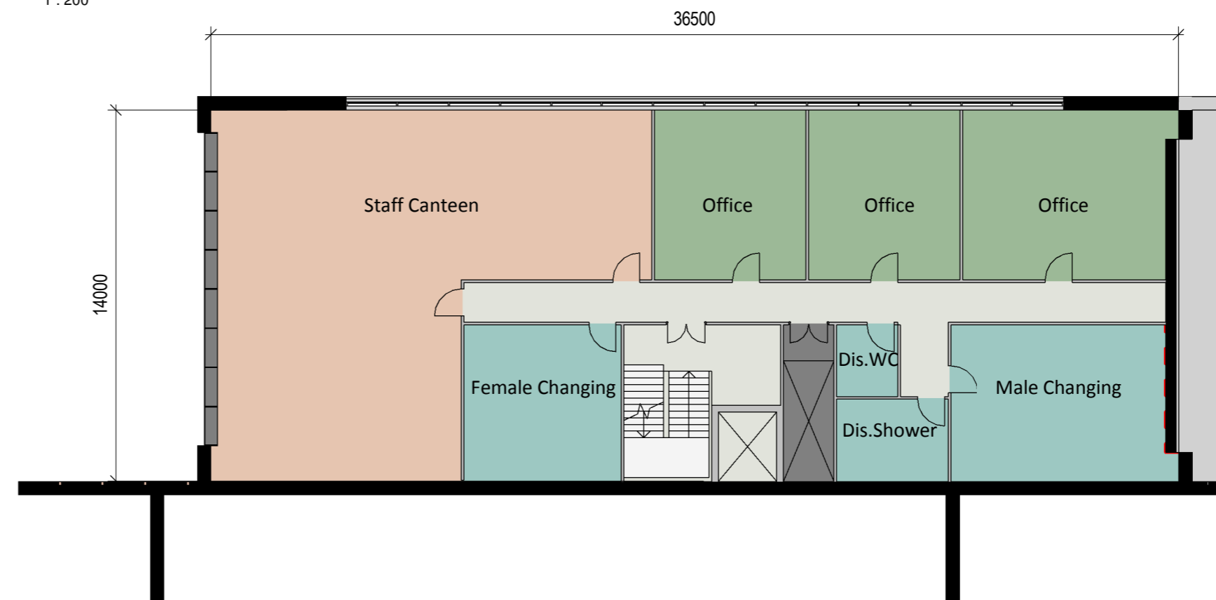
Office Plan - Level 01 1 : 200
